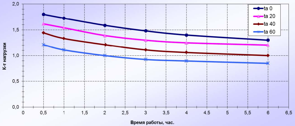
Нагрузочная характеристика ОСМ1-0,063
