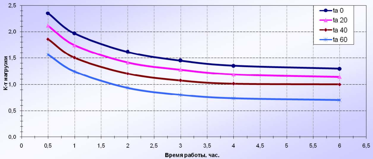
Нагрузочная характеристика ОСМ1-1,0М
