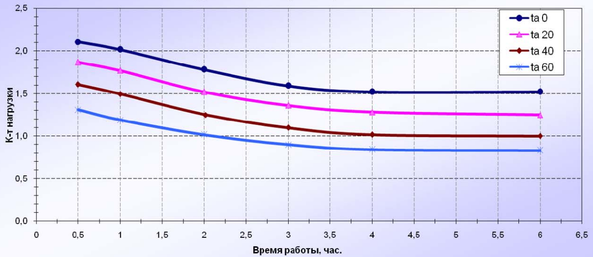
Нагрузочная характеристика ОСМ1-0,16
