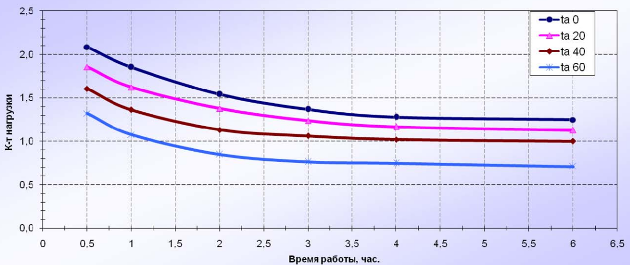
Нагрузочная характеристика ОСМ1-0,63М
