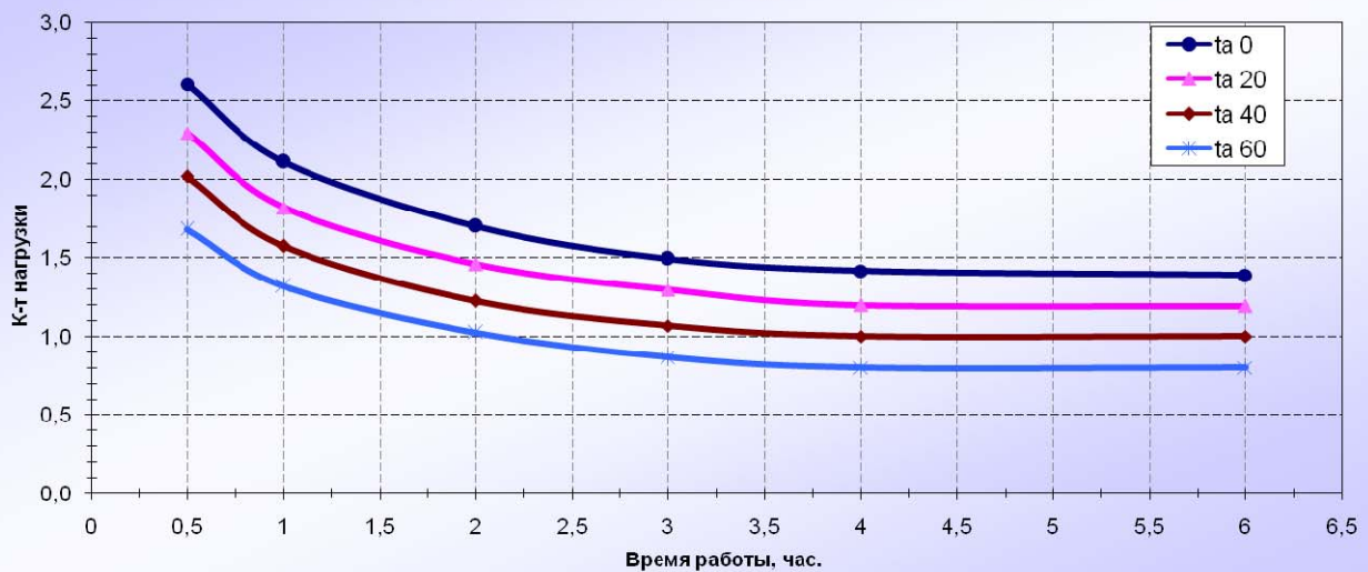
Нагрузочная характеристика ОСМ1-2,5М
