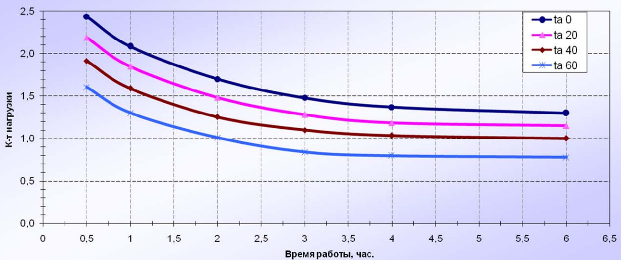
Нагрузочная характеристика ОСМ1-1,6М
