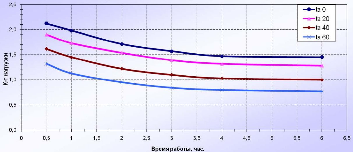
Нагрузочная характеристика ОСМ1-0,25
