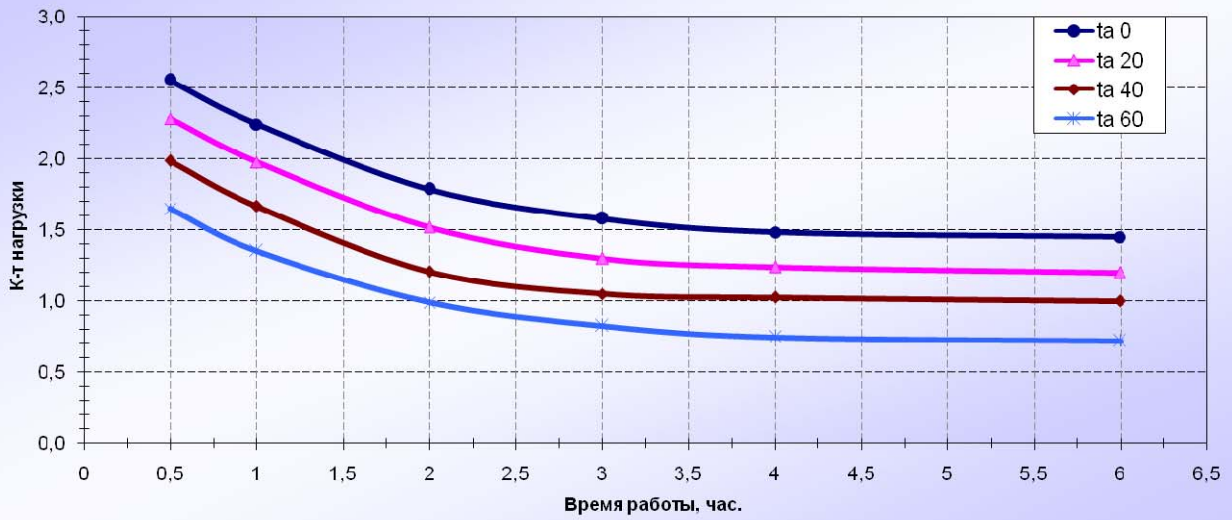
Нагрузочная характеристика ОСМ1-0,4
